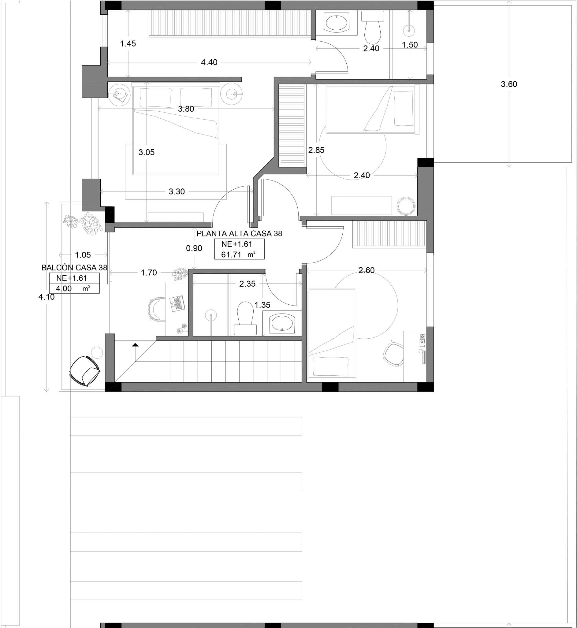
PLANTA ALTA ESCALA 1:50
