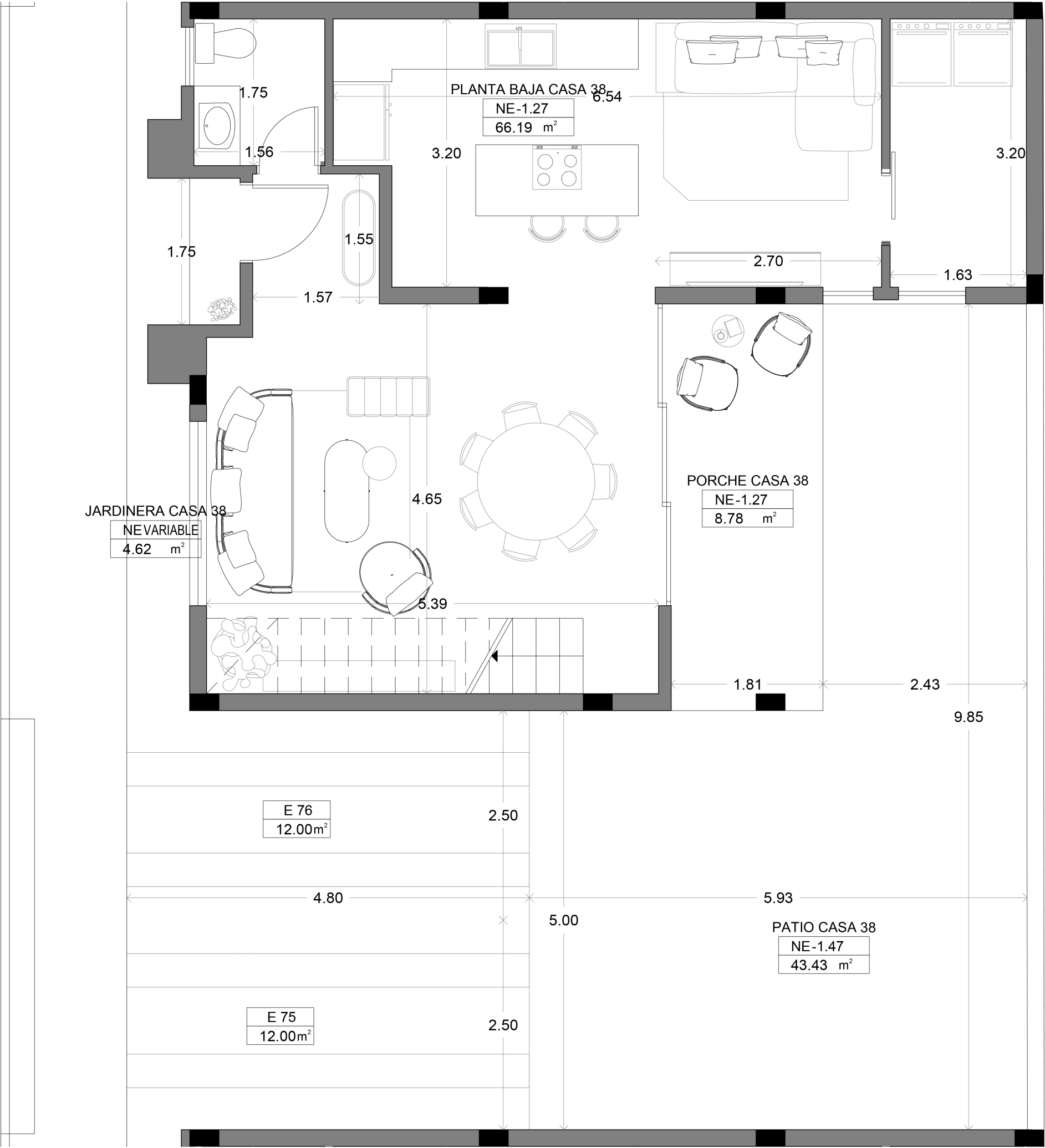
PLANTA BAJA ESCALA 1:50
